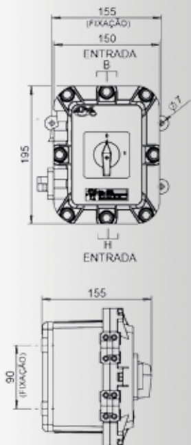
Dimensões em mm.
